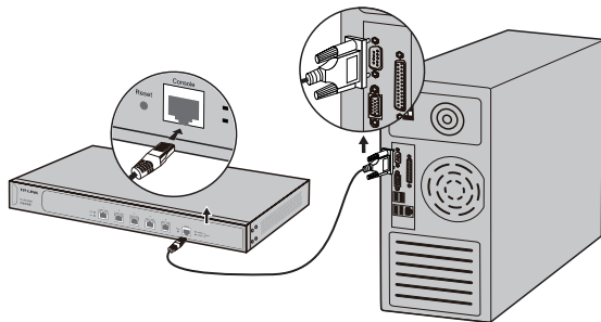
图3-2 Console端口连接示意图
